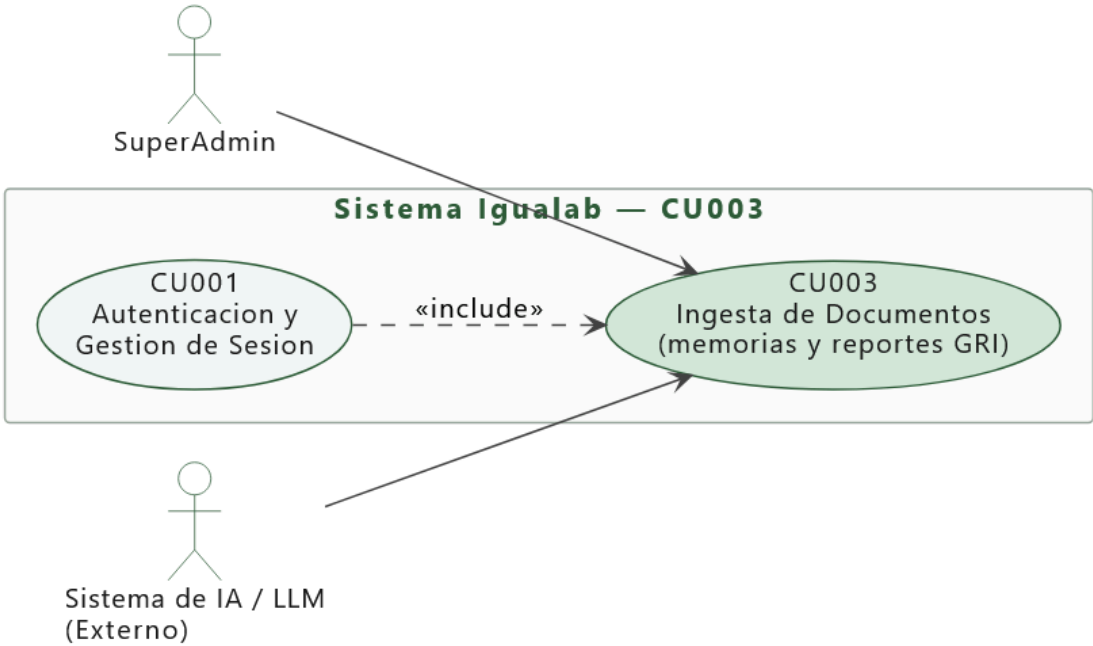
[ IMAGEN ] Diagrama de caso de uso — CU003
